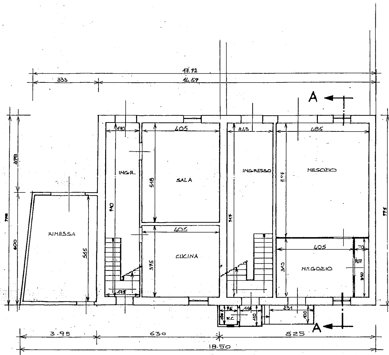
PIANTA PIANO TERRENO
