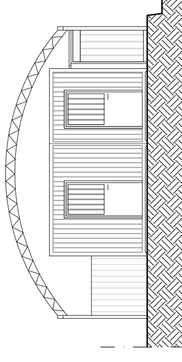
Prospetto Sud
