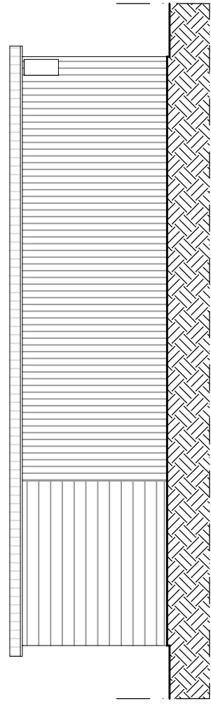
Prospetto Est
