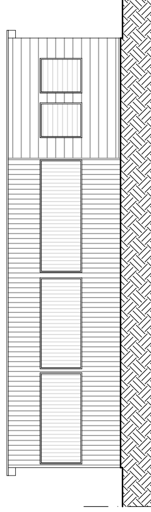
Prospetto Ovest
