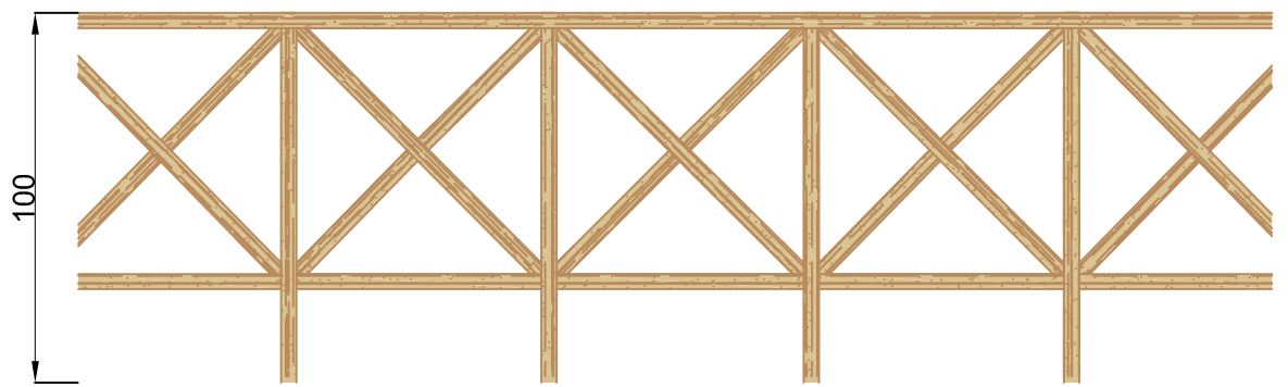
RECINZIONE IN LEGNO DIVISIONE PARCO STRADA PUBBLICA
