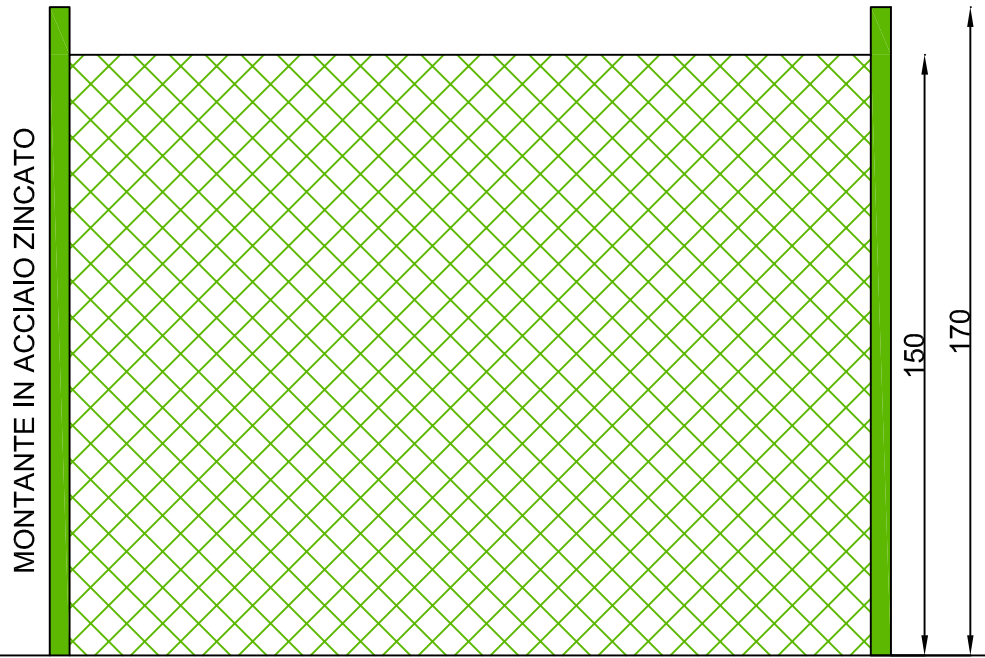
DIVISIONE STRADA PUBBLICA CON PASSO PEDONALE
